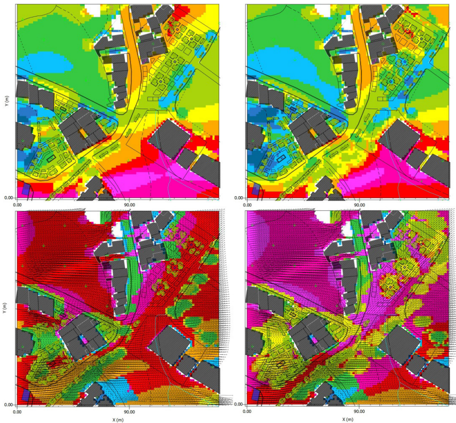
تصویر شماره ۸: بررسی شرایط آسایش، ردیف بالا ساعت ۱۲:۰۰ ظهر، ردیف پایین ۱۴:۰۹ بعدازظهر، سمت راست طرح پیشنهادی، سمت چپ حالت وضع موجود
