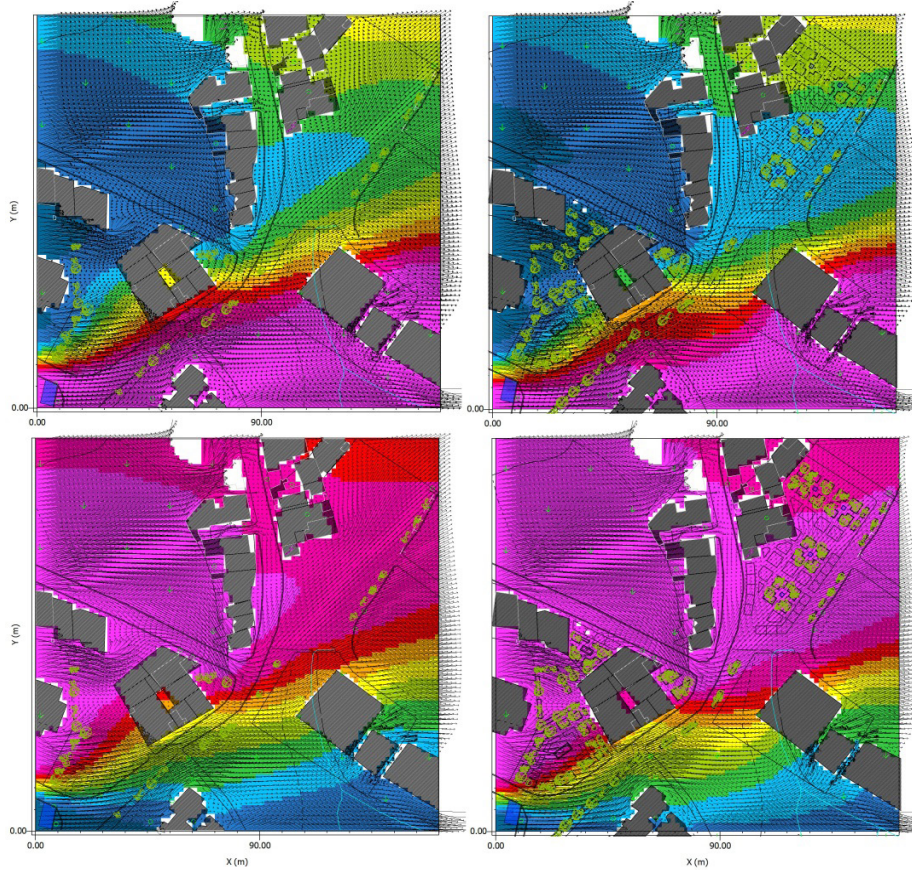
تصویر شماره ۷: رطوبت نسبی، ردیف بالا ساعت ۱۲:۰۰ ظهر، ردیف پایین ۱۴:۰۹ بعدازظهر، سمت راست طرح پیشنهادی، سمت چپ حالت وضع موجود
