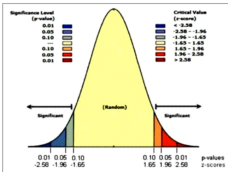
نمودار شماره ۱- مقادیر Z و P روی نمودار توزیع نرمال
